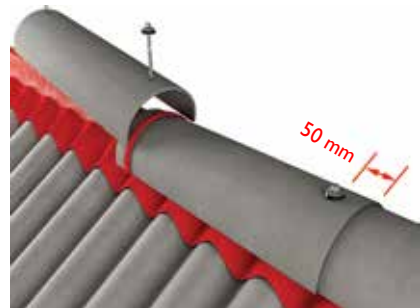
rys. 35. Sposób montażu gąsiora konikalnego.
