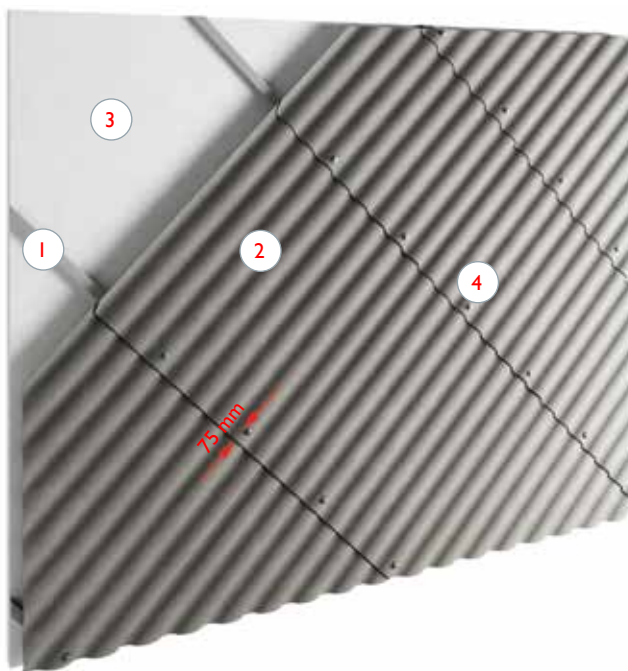
rys.53. Montaż płyt na elewacji/ścianie ukośnie z zakładem podłużnym (na jedną falę) i zakładem poprzecznym (150 mm). 1 - łąty pod wybranym kątem (ukośnie) do poziomemu gruntu 2 - płyta EuroFala mocowana z zakładem podłużnym (na jedną falę) i zakładem poprzecznym (150 mm) 3 - istniejąca wcześniej elewacja/ściana budynku 4 - punkty mocowania płyt - dla płyt B59 na szczytach 2 i 6 fali, dla płyt B65 na szczytach 2 i 5 fali
