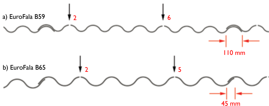
rys. 16a. Miejsca wykonania otworów montażowych dla krycia rozpoczętego z lewej strony połaci dachowej - EuroFala B59. rys. 16b. Miejsca wykonania otworów montażowych dla krycia rozpoczętego z lewej strony połaci dachowej - EuroFala B65.
