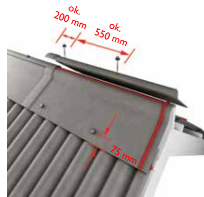
rys. 36. Sposób montażu gąsiora zawiasowego płaskiego.
