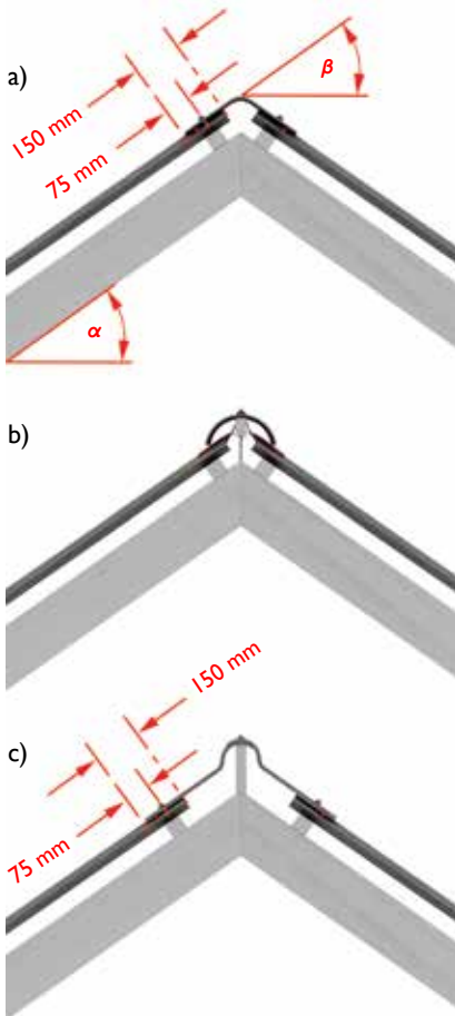
rys.34. Sposób wykończenia kalenicy: a - gąsioro kątowym b - gąsioro konikalnym / stożkowym c - gąsioro zawiasowym płaskim
