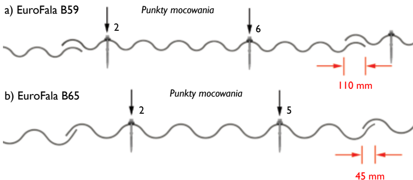
rys.24a. Punkty mocowań płyty EuroFala B59 na połaci dachowej znajdują się na szczycie 2 i 6 fali. Rysunek przedstawia krycie połaci dachowej od lewej do prawej strony.
