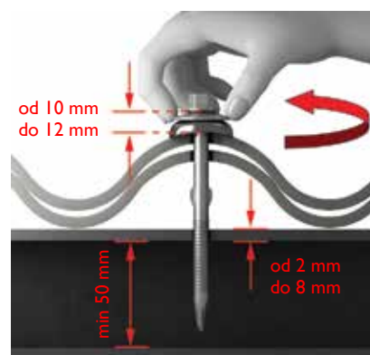
rys.27. System montażowy Quick Fix do konstrukcji stalowej przykręcony poprawnie. Prawidłowość przykręcenia systemu montażowego ocenia się wizualnie oraz próbując okręcić stalową podkładką dociskową wokół osi wkrętu. Jeżeli nie jest to możliwe to znaczy, że system montażowy jest przykręcony zbyt mocno i musi zostać poluzowany. Można go stosować przy grubości stali od 2 mm do 8 mm. Odległość wewnętrzna pomiędzy ściankami płatwi stalowych powinna wynosić minimum 50 mm. Systemy montażowe Quick Fix do konstrukcji stalowej zostały wyposażone w dodatkowy frez na ostrzu wiertącym. Rozwiera on wstępny otwór montażowy w płycie, a następnie wyłamuje się podczas wiercenia w konstrukcji stalowej.
