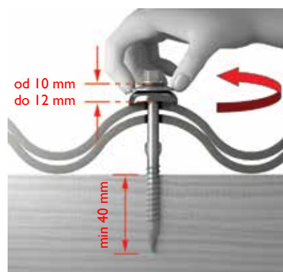
rys.26. System montażowy Quick Fix do konstrukcji drewnianej przykręcony poprawnie. Prawidłowość przykręcenia systemu montażowego ocenia się wizualnie oraz próbując okręcić stalową podkładką dociskową wokół osi wkrętu. Jeżeli nie jest to możliwe to znaczy, że system montażowy jest przykręcony zbyt mocno i musi zostać poluzowany. Wkręt musi być wkręcony do łąty/płatwi na głębokość min. 40 mm.
