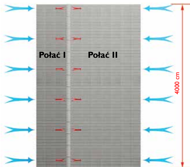
rys.12. Rysunek do przykładu obliczenia powierzchni otworów wentylacyjnych - rzut i przekrój dachu. Niebieskie strzałki - powierzchnia otworów wentylacyjnych wlotowych w okapie. Czerwone strzałki - powierzchnia otworów wentylacyjnych wylotowych w kalenicy.
