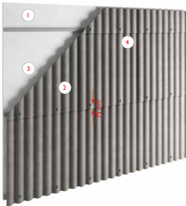
rys.54. Montaż płyt na elewacji/ścianie pionowa z zakładem podłużnym (na jedną falę) i zakładem poprzecznym (150 mm) 1 - łąty równoległe do poziomu gruntu 2 - płyta EuroFala mocowana z zakładem podłużnym (na jedną falę) i zakładem poprzecznym (150 mm) 3 - istniejąca wcześniej elewacja/ściana budynku 4 - punkty mocowania płyt - dla płyt B59 na szczytach 2 i 6 fali, dla płyt B65 na szczytach 2 i 5 fali
