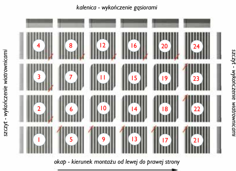
rys. 23. Prawidłowa kolejność układania płyt EuroFala NO/WO zgodnie z numeracją od 1 do 21.
